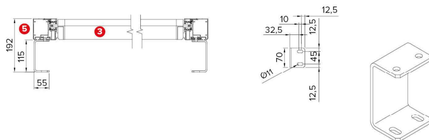
Dettaglio frangivento . Wind-break detail 088-930
