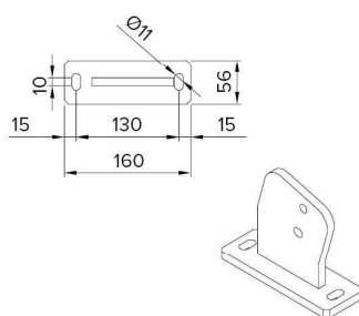
Piede a terra . Foot
